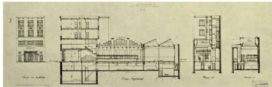
Façades et coupes, 1932.
